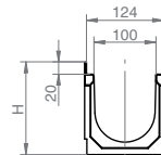
PDGS 150 techn. Maße
