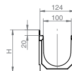
PDGS 150 techn. Maße
