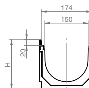
PDGS 200 techn. Maße
