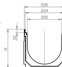
PDGS 200 techn. Maße
