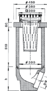
ohne Geruchsverschluss
