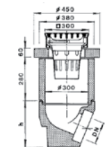
ohne Geruchsverschluss
