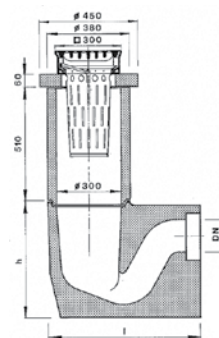
mit Geruchsverschluss
