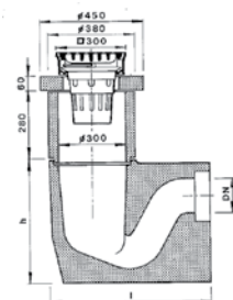
mit Geruchsverschluss
