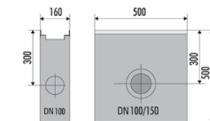
Einlaufkasten FFIX8053
