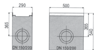
Einlaufkasten
