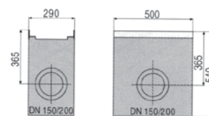
Einlaufkasten
