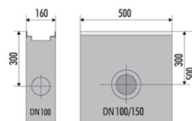
Einlaufkasten
