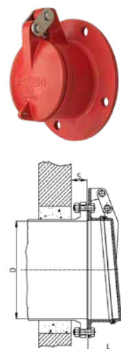
Flanschverbindung (Flanschtyp: PN10)
