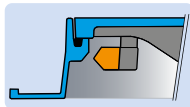
Abb. 9: Federstab verbogen: Position zu weit innen, Deckel ist lose
