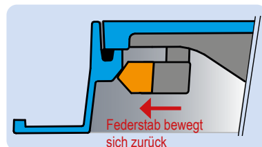
Abb. 7: Federstab in richtiger Position nach dem Schließen des Deckels (korrekt fixiert)
