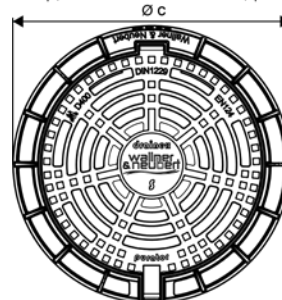
Variante hochziehbarer Gussrahmen
