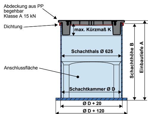
Einbauschema mit Kunststoffabdeckung Klasse A 15 begehbar
