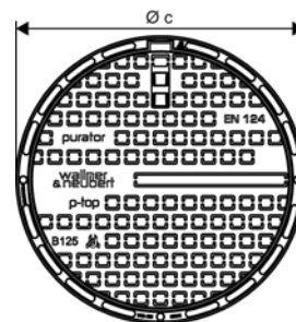
Variante Beton-Gussrahmen
