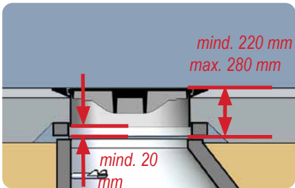
Einbau DRAINEX Niveau mit Adaptring
