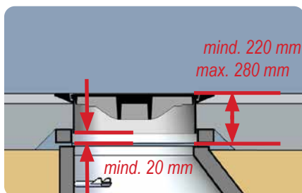
Einbau F-TOP Niveau mit Adapting
