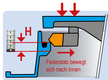
Abb. 6: Federstab im Schnitt in richtiger Position vor dem Schließen des Deckels
