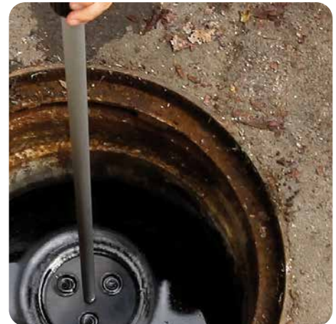
Sichtkontrolle der Abscheideroberfläche bei einem SeparateurBLUE
