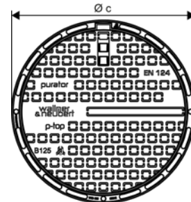
Variante Beton-Gussrahmen
