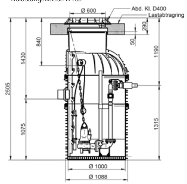
Belastungsklasse D400
