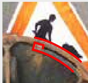
richtige horizontale Pos.: Federstabbogen etwa parallel zur Deckelrundung, Vorderkante des Federstabes ca. 8 mm über Rahmeninnenkante
