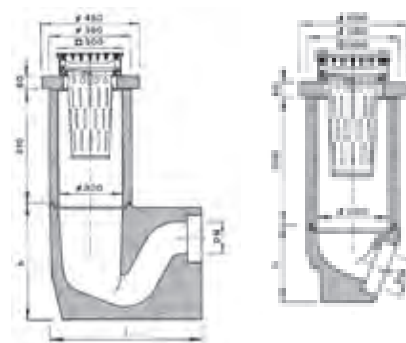
mit Geruchsverschluss
