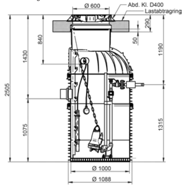
Belastungsklasse D400
