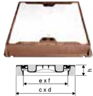
Bild zeigt Gussrahmen Schnitt BEGE-Rahmen
