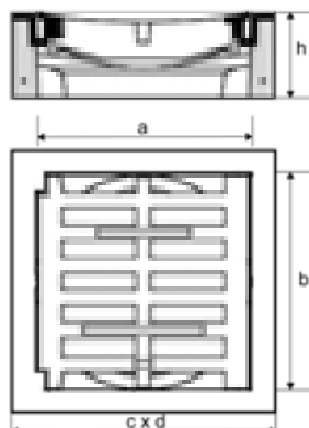
Ausführung Rinnenform
