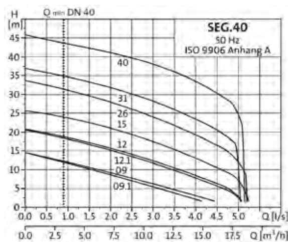
Typen SEG.40
