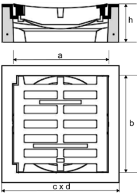
Ausführung Rinnenform
