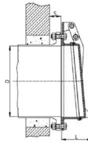
Flanschverbindung (Flanshtyp: PN10)
