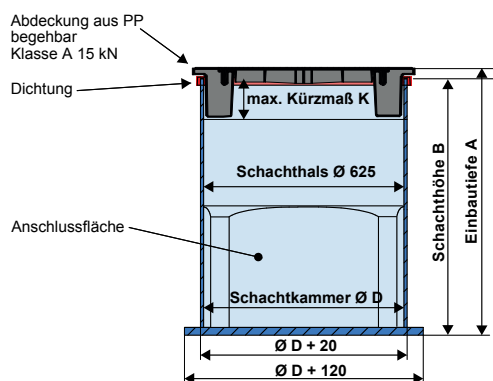
Einbauschema mit Kunststoffabdeckung Klasse A 15 begehbar
