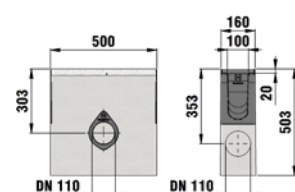
Einlaufkasten
