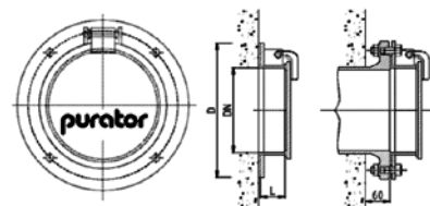
Wandbefestigung mit Dübel Flanschverbindung (Flanshtyp: PN10)
